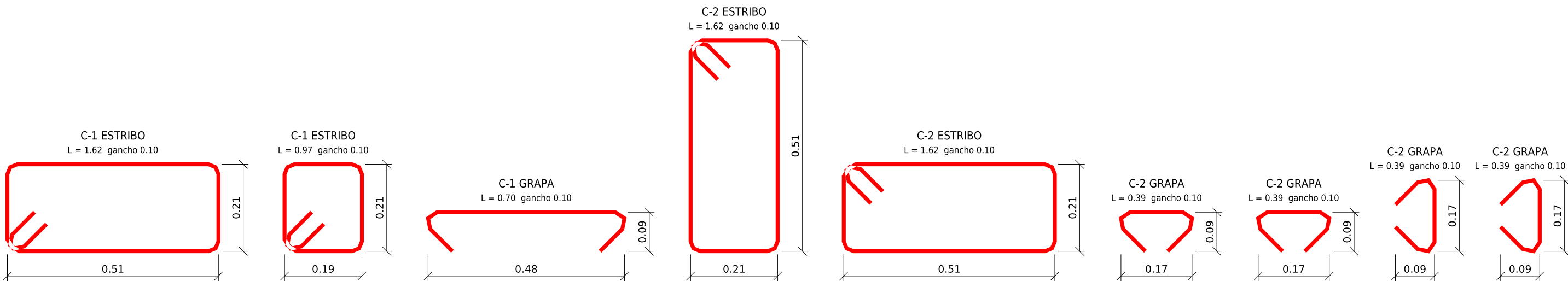
DETALLE DE ESTRIBOS Y GRAPAS (juego típico, medidas exteriores del modelo) ESC. 1:10
