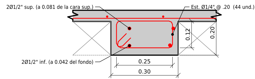
DETALLE 5-5 VIGA CHATA VCH
