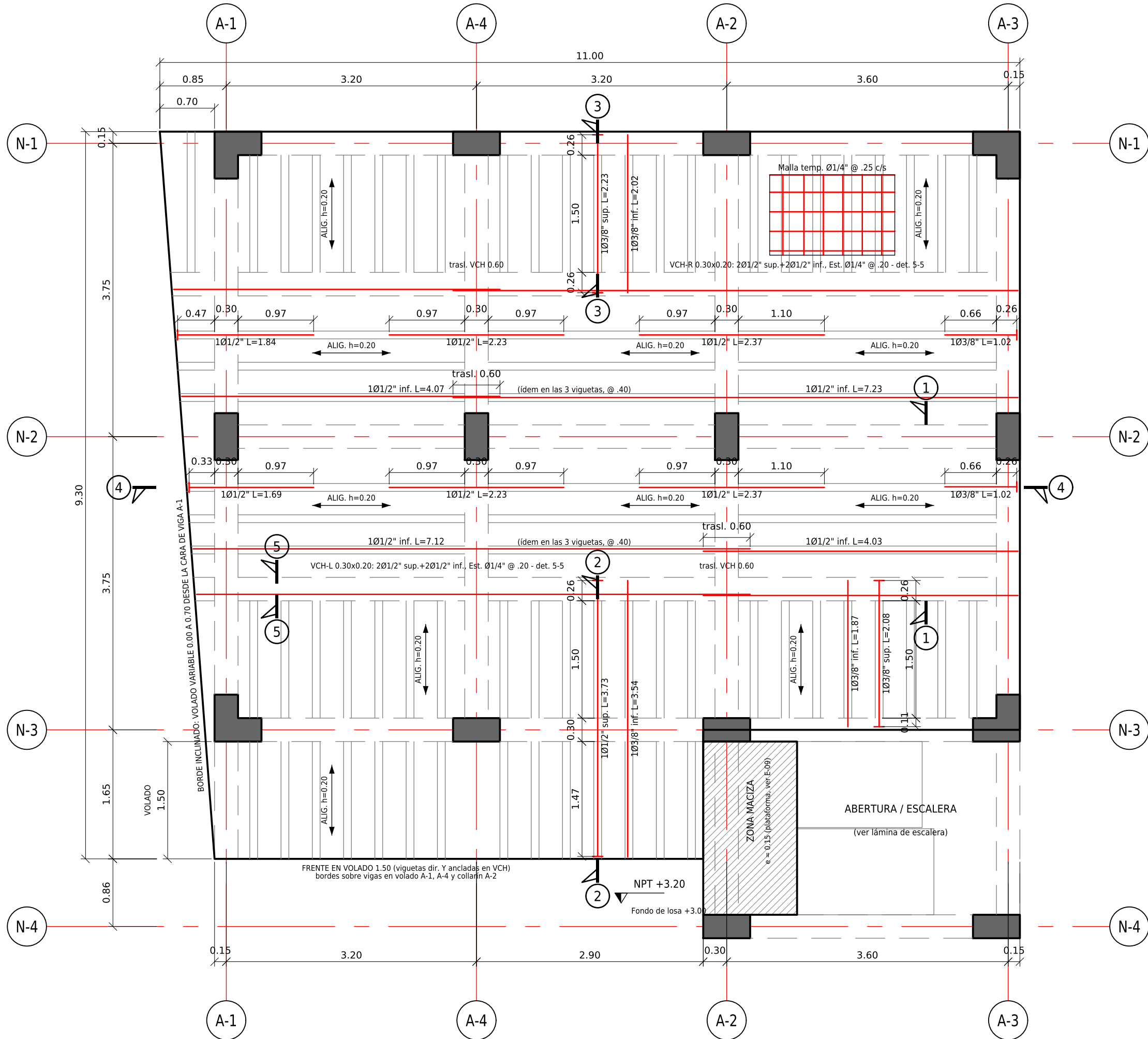
PLANTA DE LOSA ALIGERADA - NIVEL 2 (NPT +3.20)
