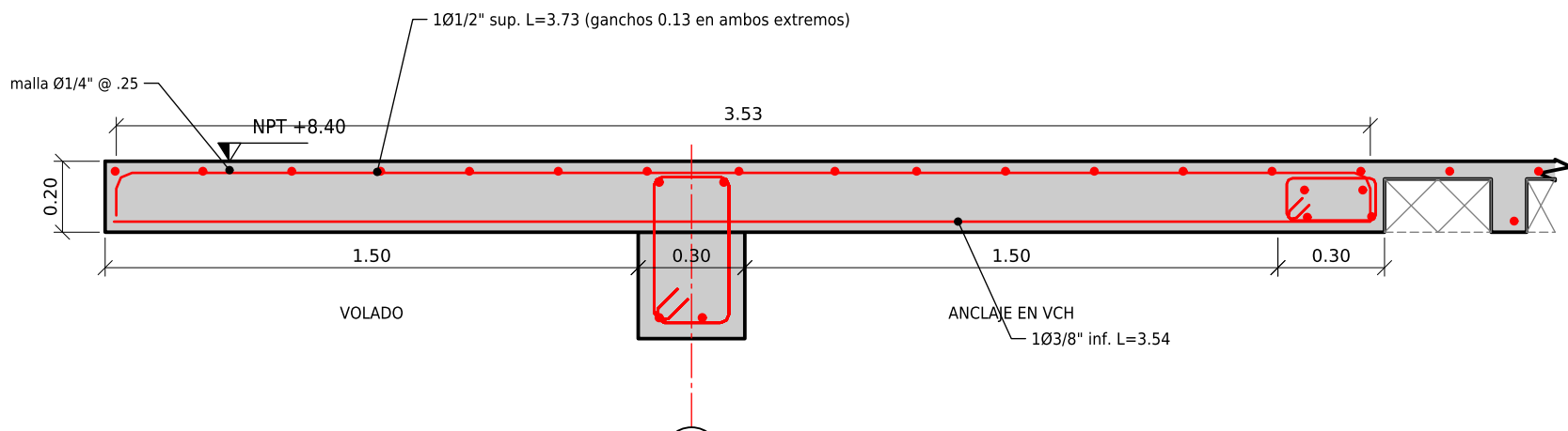
CORTE 2-2 VOLADO LADO N-4 Y VCH
