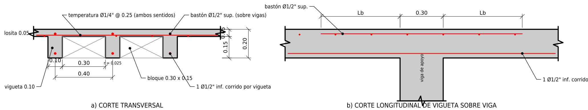
DETALLE DE ALIGERADO
