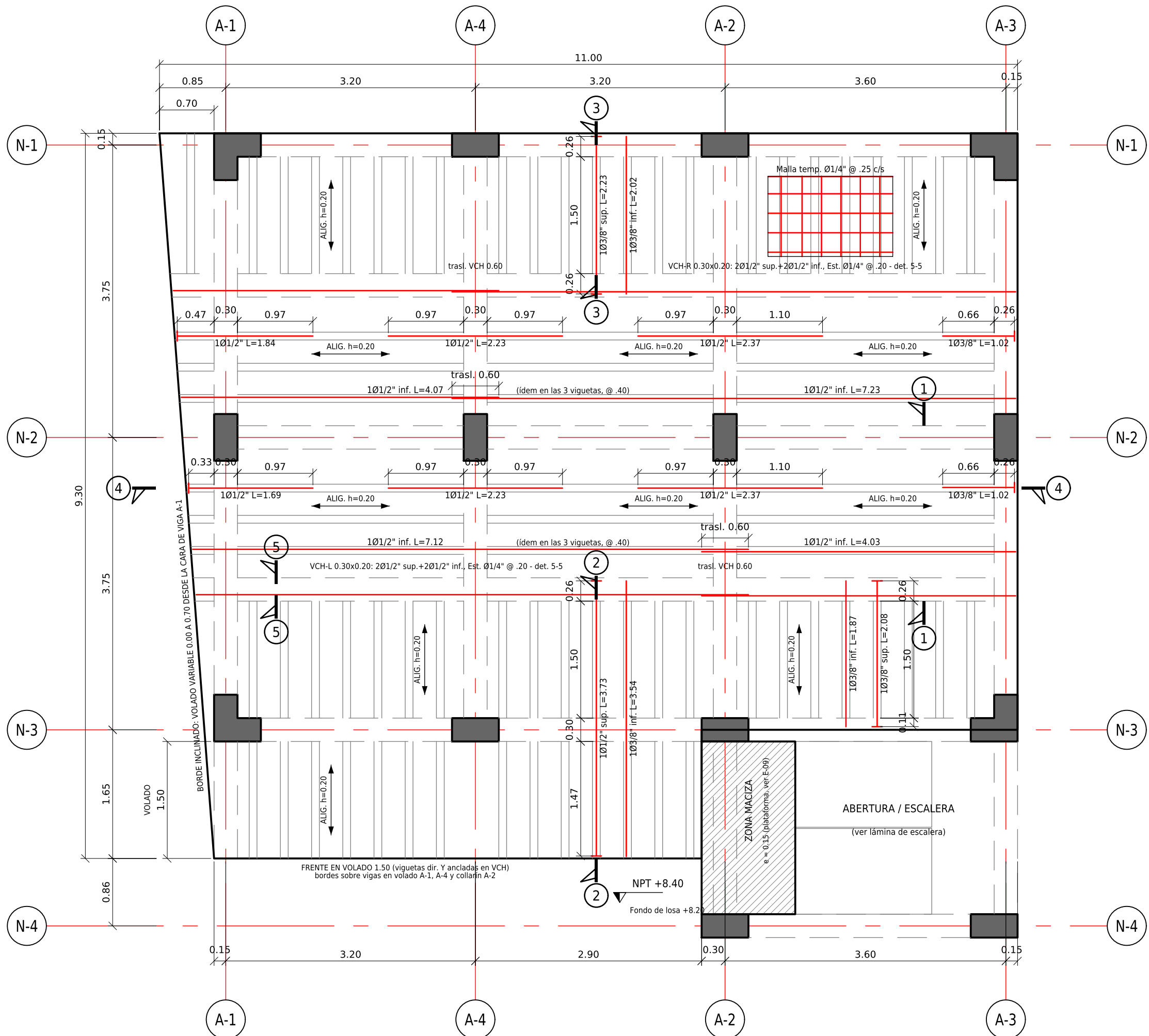
PLANTA DE LOSA ALIGERADA - NIVEL 4 (NPT +8.40)
