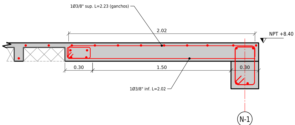
CORTE 3-3 BORDE N-1 Y VCH
