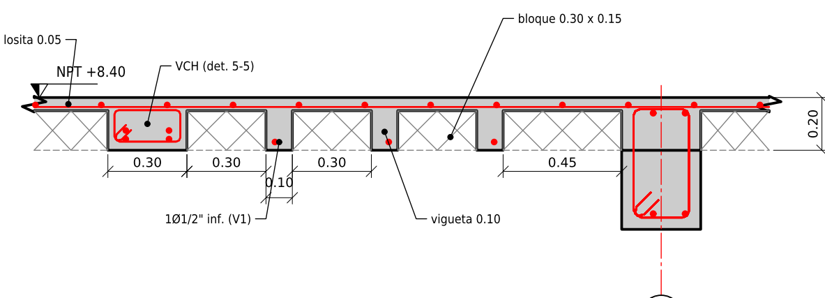
CORTE 1-1 ALIGERADO TÍPICO
