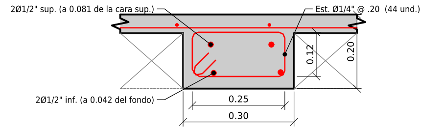
DETALLE 5-5 VIGA CHATA VCH
