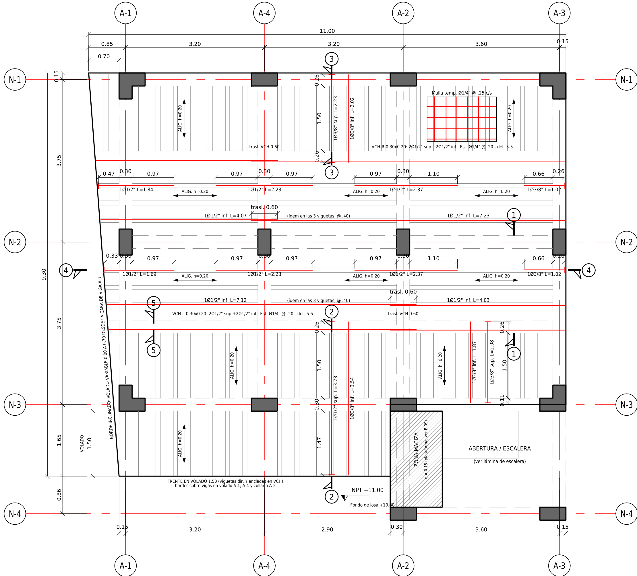
PLANTA DE LOSA ALIGERADA - NIVEL 5 (NPT +11.00)
