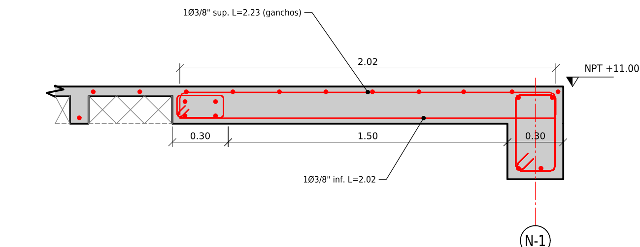
CORTE 3-3 BORDE N-1 Y VCH
