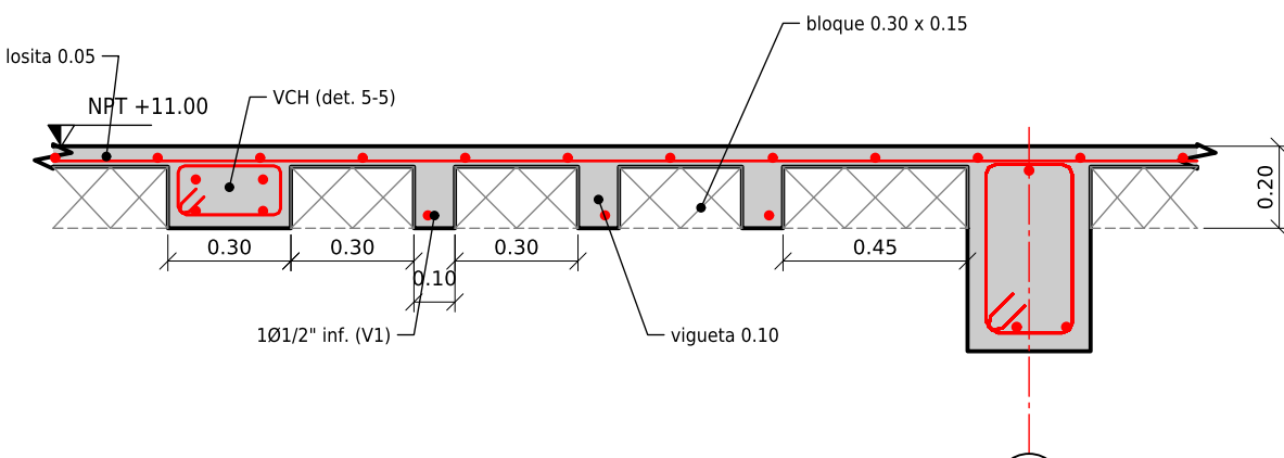
CORTE 1-1 ALIGERADO TÍPICO
