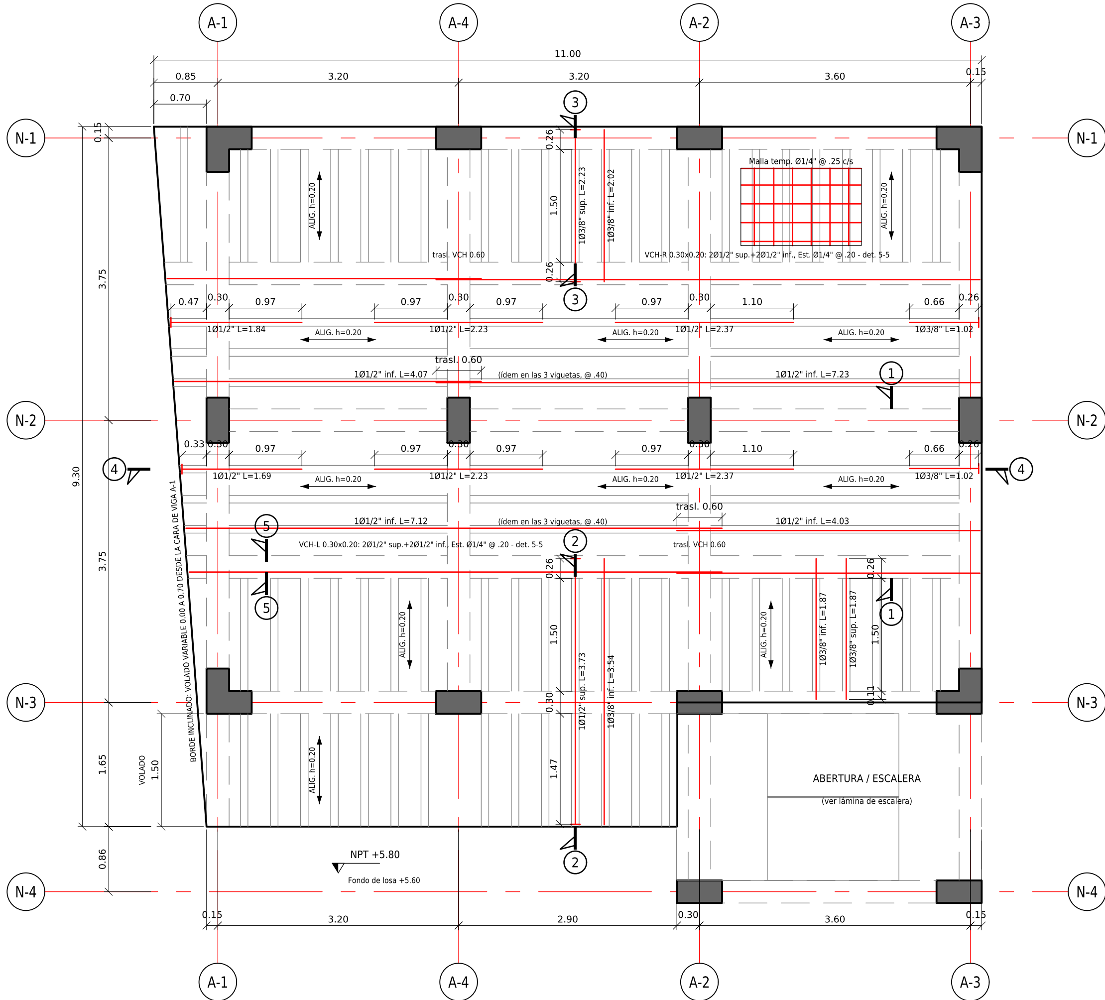
PLANTA DE LOSA ALIGERADA - NIVEL 3 (NPT +5.80)
