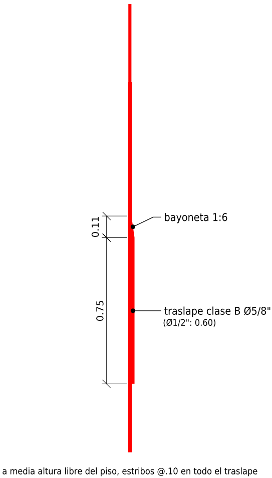
DETALLE DE TRASLAPE ESC. 1:20
