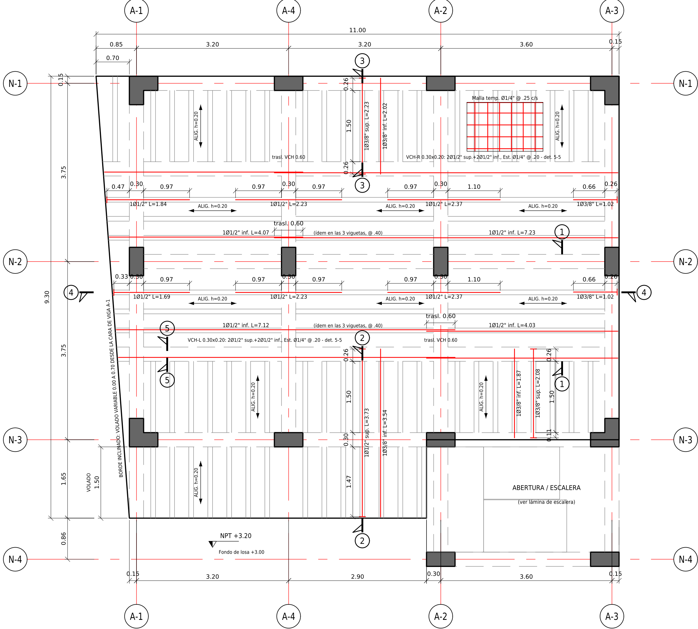
PLANTA DE LOSA ALIGERADA - NIVEL 2 (NPT +3.20) ESC. 1:50
