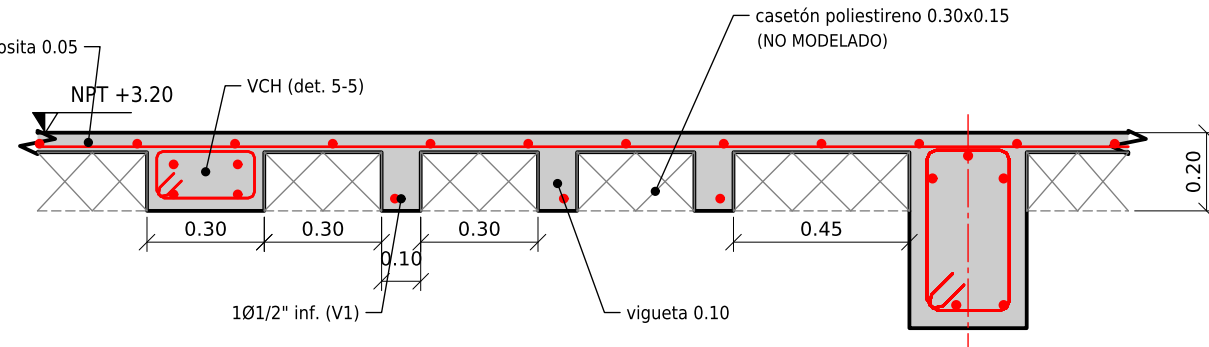
CORTE 1-1 ALIGERADO TÍPICO ESC. 1:20
