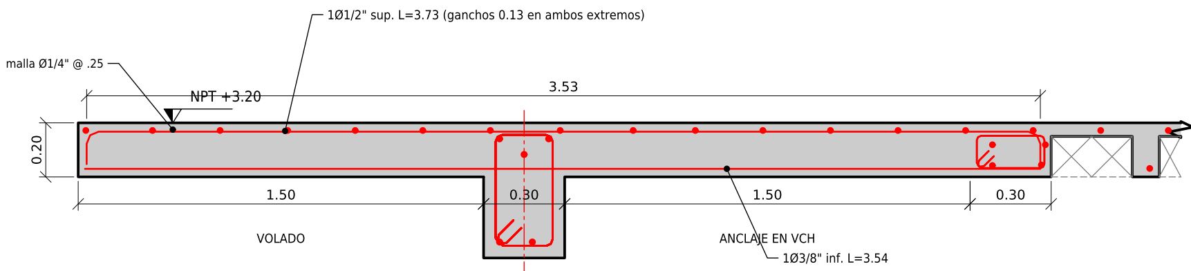
CORTE 2-2 VOLADO LADO N-4 Y VCH ESC. 1:20
