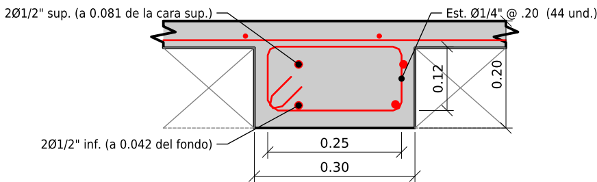
DETALLE 5-5 VIGA CHATA VCH ESC. 1:10
