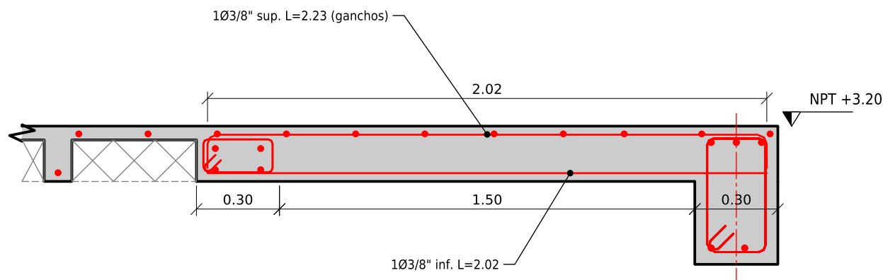
CORTE 3-3 BORDE N-1 Y VCH ESC. 1:20
