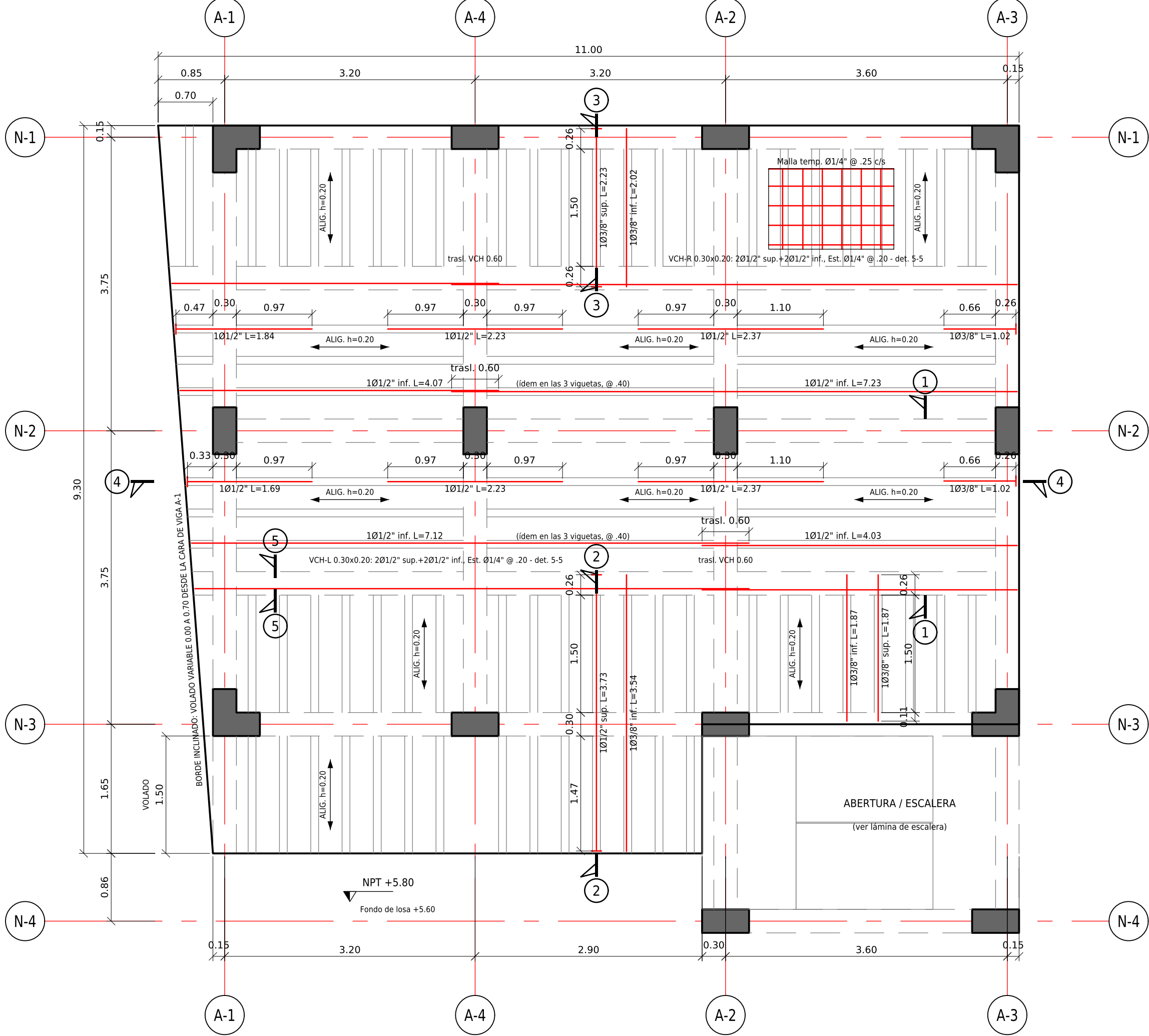
PLANTA DE LOSA ALIGERADA - NIVEL 3 (NPT +5.80) ESC. 1:50
