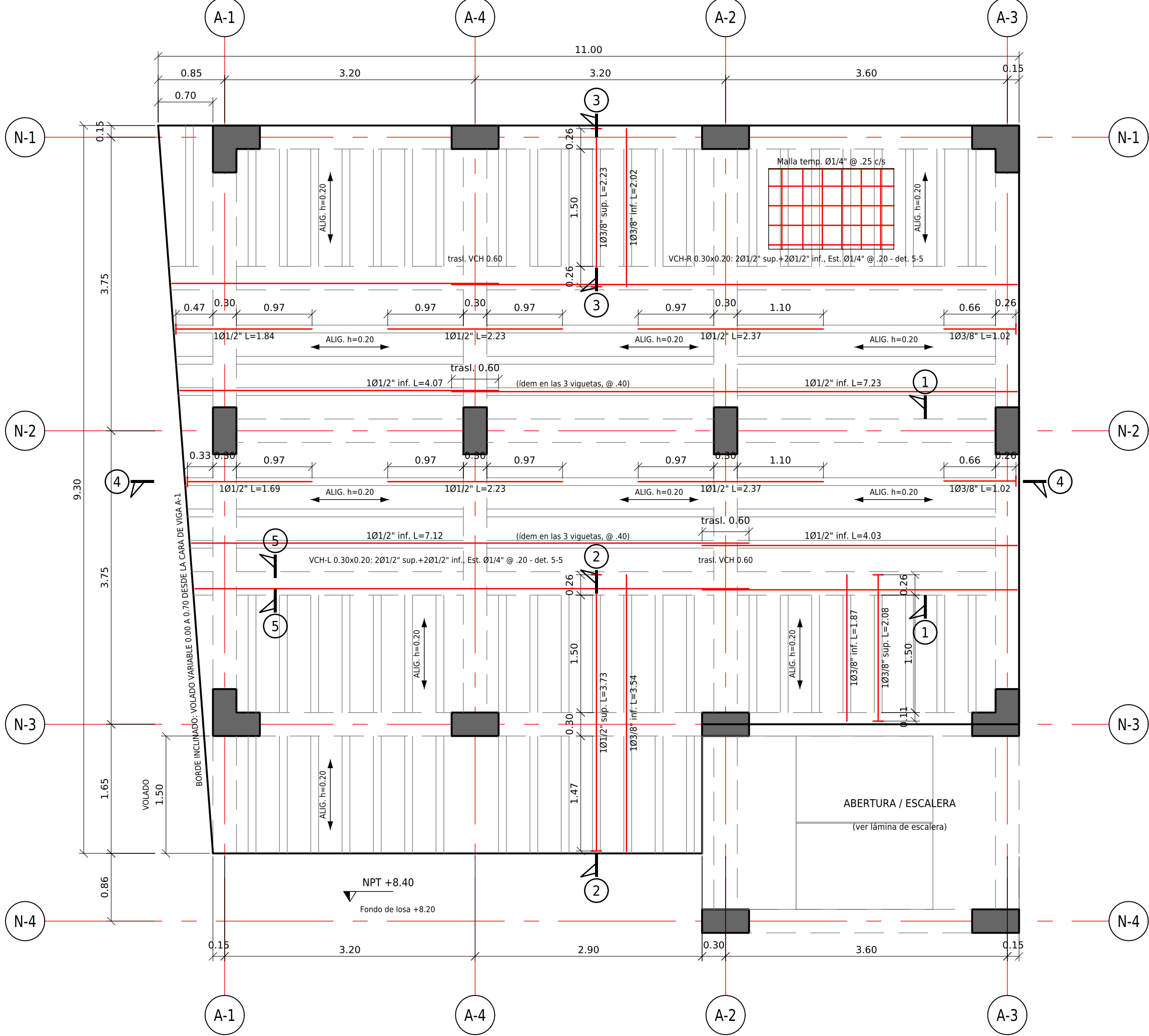
PLANTA DE LOSA ALIGERADA - NIVEL 4 (NPT +8.40) ESC. 1:50
