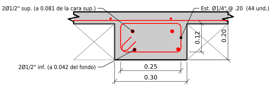
DETALLE 5-5 VIGA CHATA VCH ESC. 1:10
