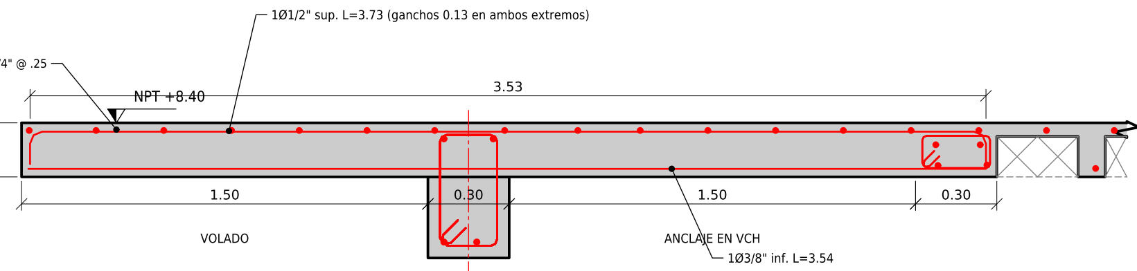
CORTE 2-2 VOLADO LADO N-4 Y VCH ESC. 1:20
