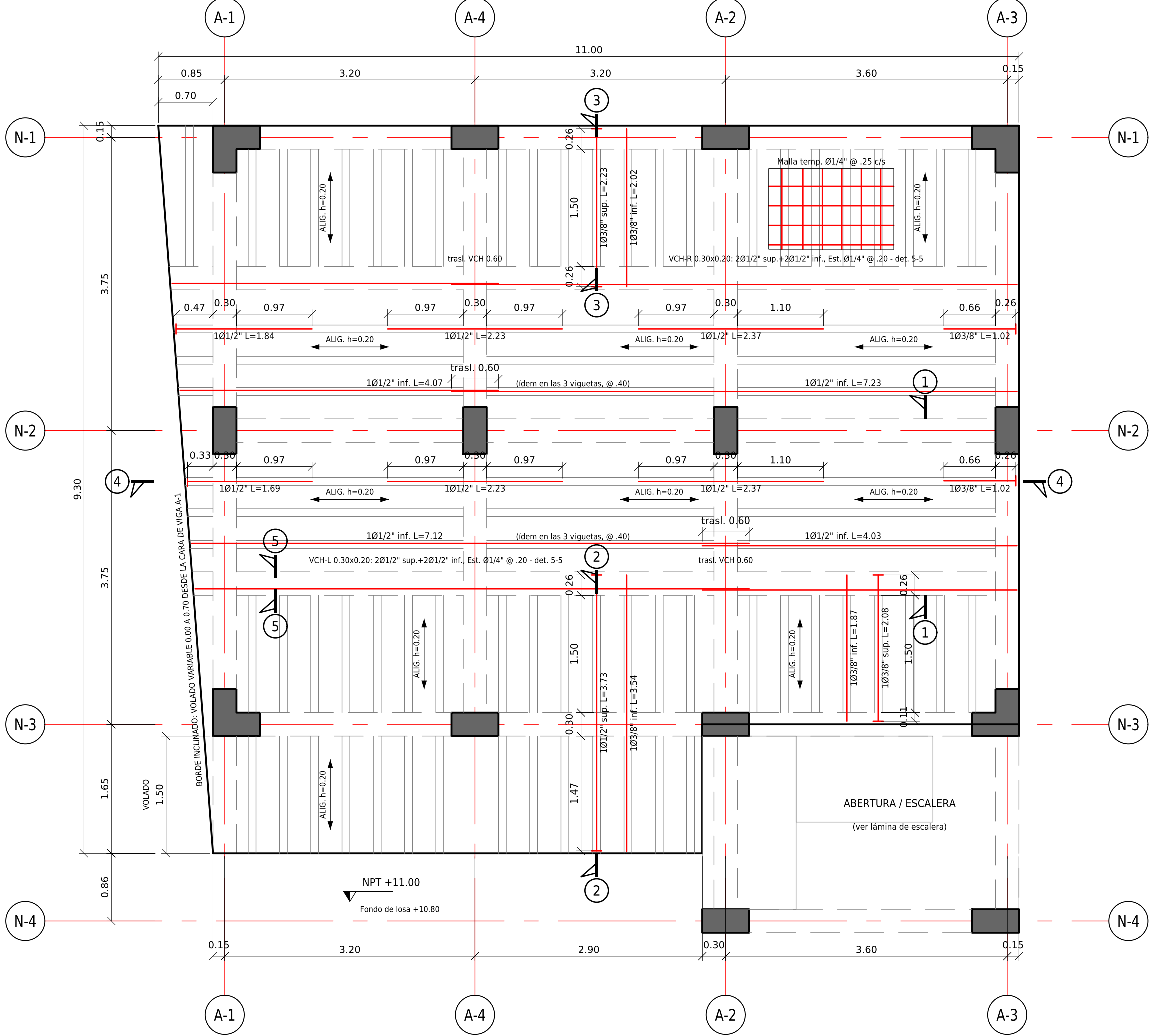
PLANTA DE LOSA ALIGERADA - NIVEL 5 (NPT +11.00) ESC. 1:50
