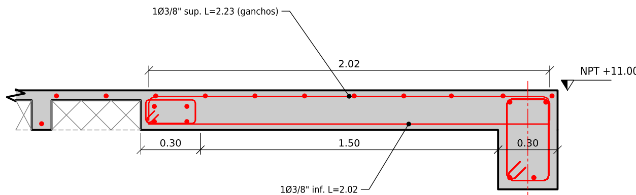
CORTE 3-3 BORDE N-1 Y VCH ESC. 1:20
