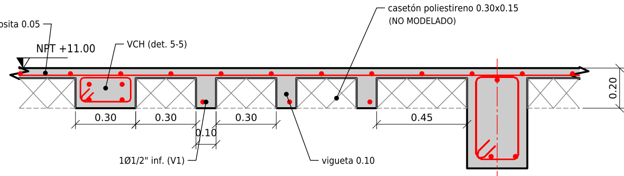
CORTE 1-1 ALIGERADO TÍPICO ESC. 1:20
