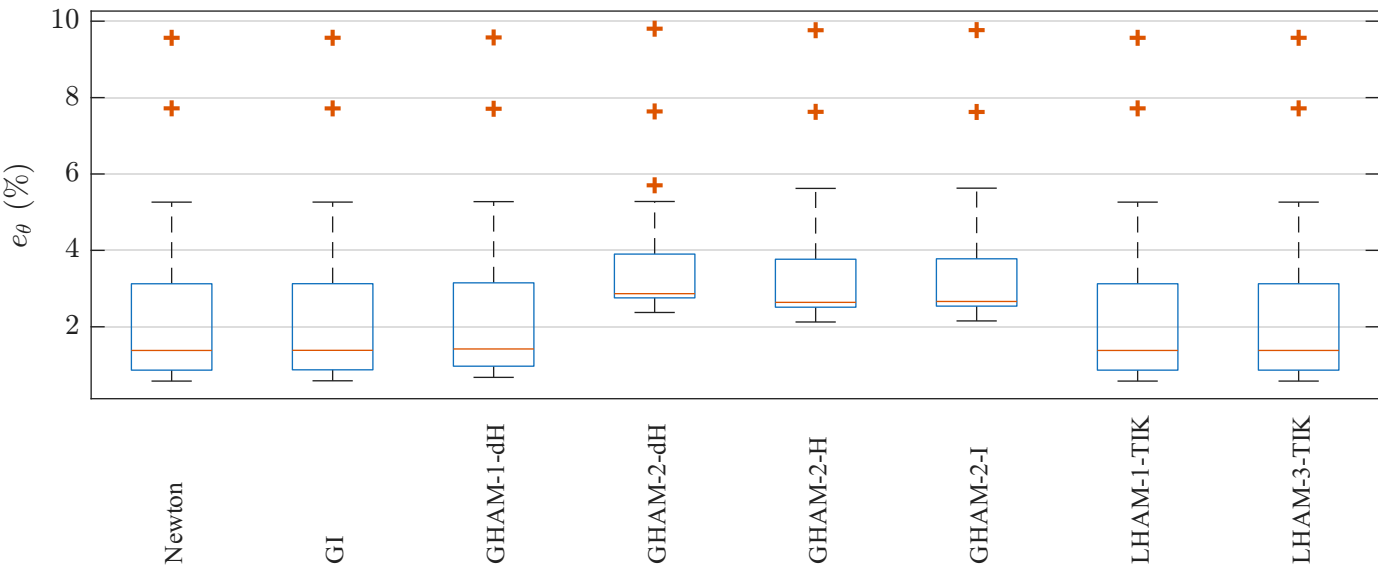
FSM Parametrization: Monte Carlo Final Parameter Error
