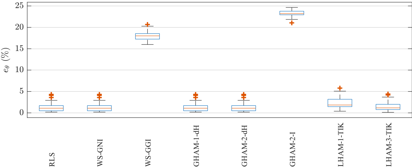
PL Parametrization: Monte Carlo Final Parameter Error
