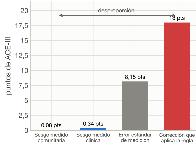
a · la regla corrige un sesgo 50 a 200 veces menor
