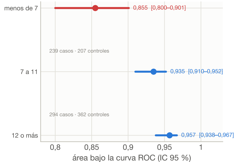
b · lo que ningún corte iguala: discriminar
