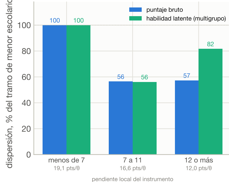
c · el puntaje se estrecha más que la habilidad
