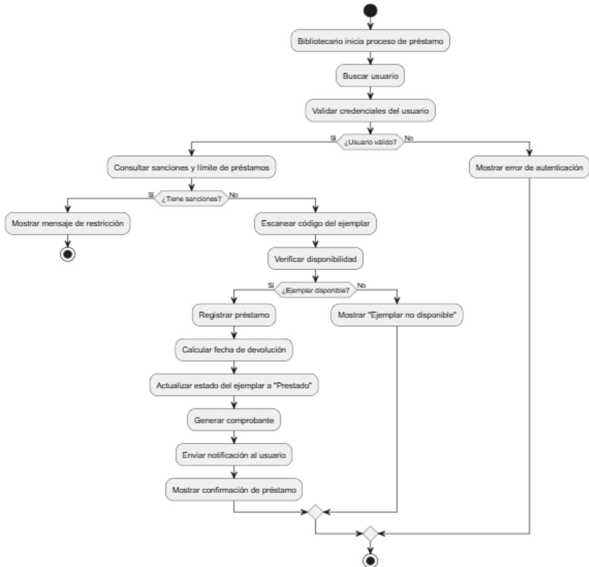
Diagrama de Actividad - Registro de Préstamo
