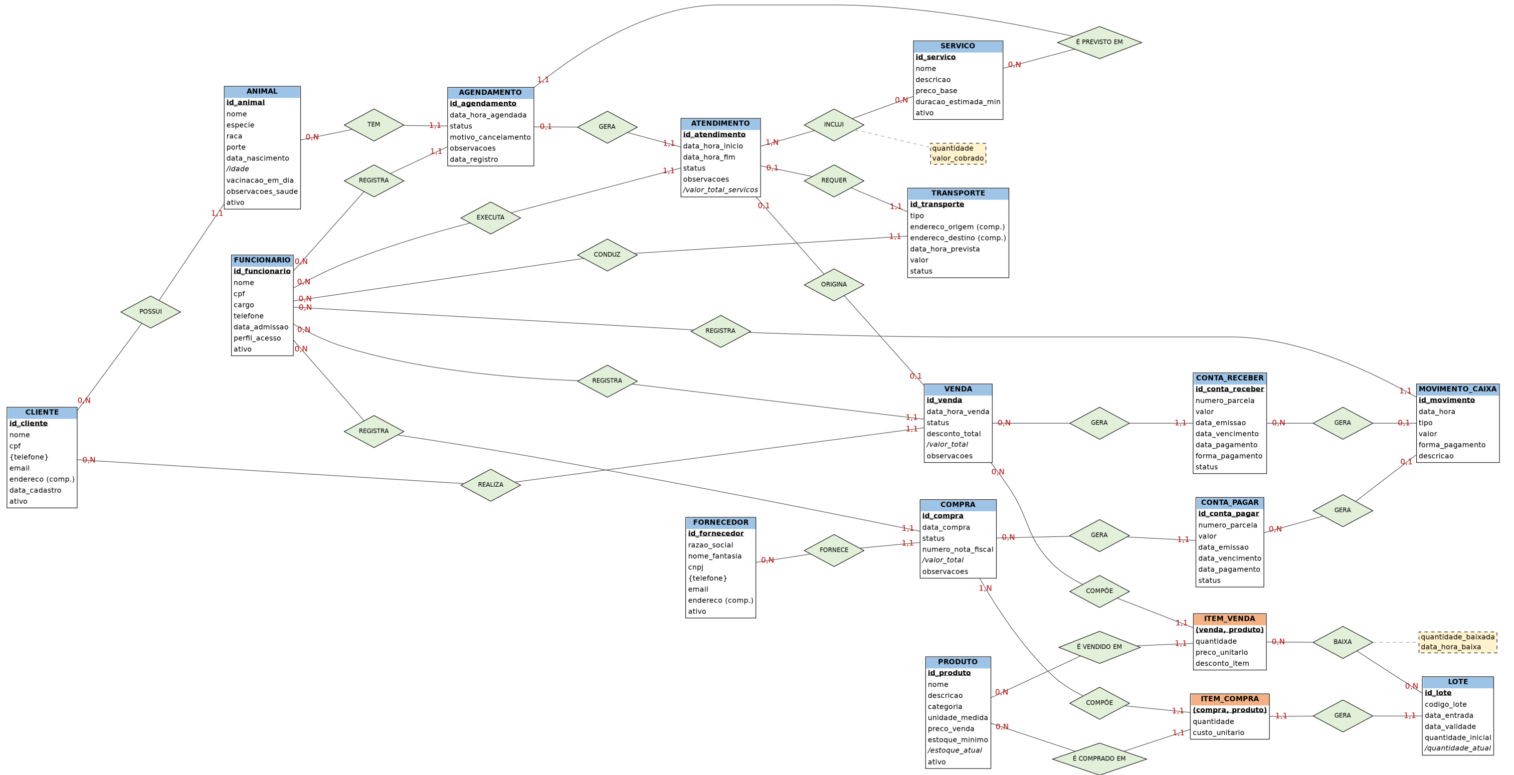
Figura 2 - Diagrama Entidade-Relacionamento (DER) conceitual. Arquivos em imagens/der_petshop.png e .svg
