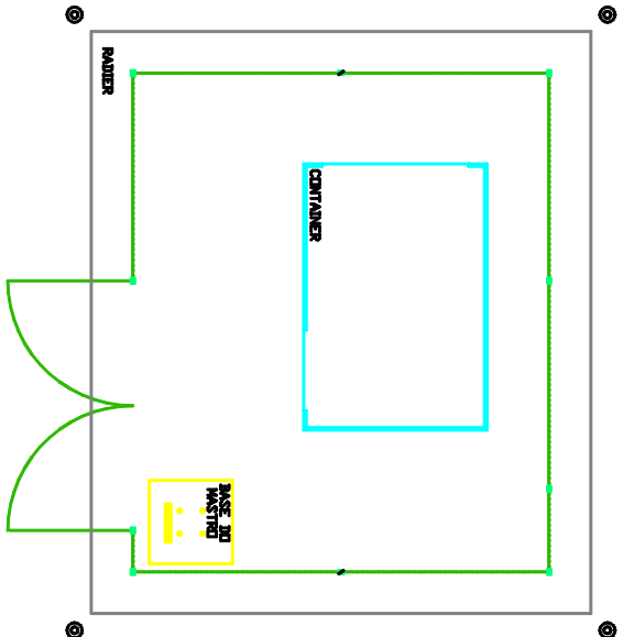
especificações da malha na folha 0024-03-01/03
