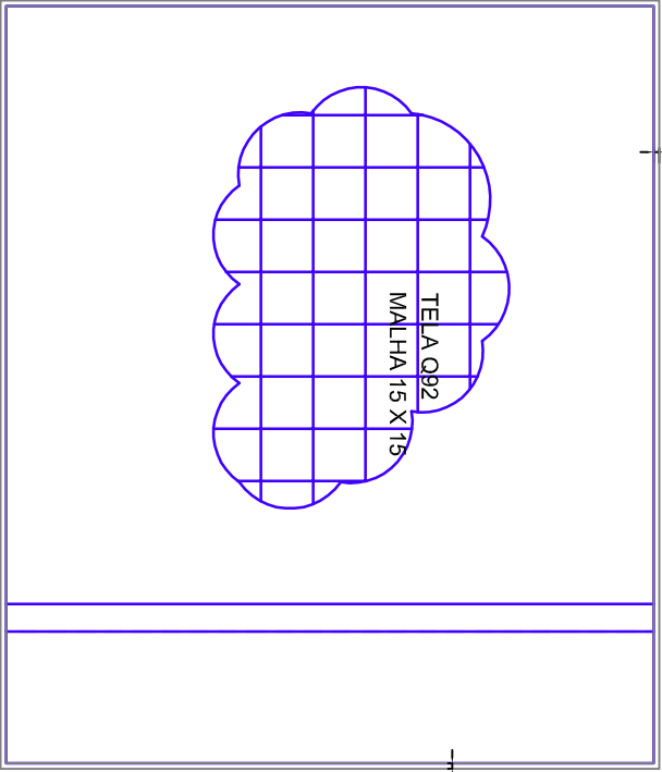
ARMADURA INFERIOR
