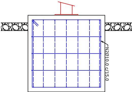
CORTE 2 - 2 ESC.: 1 : 25
