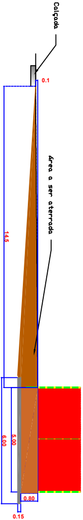
CORTE A -A Sem Escala
