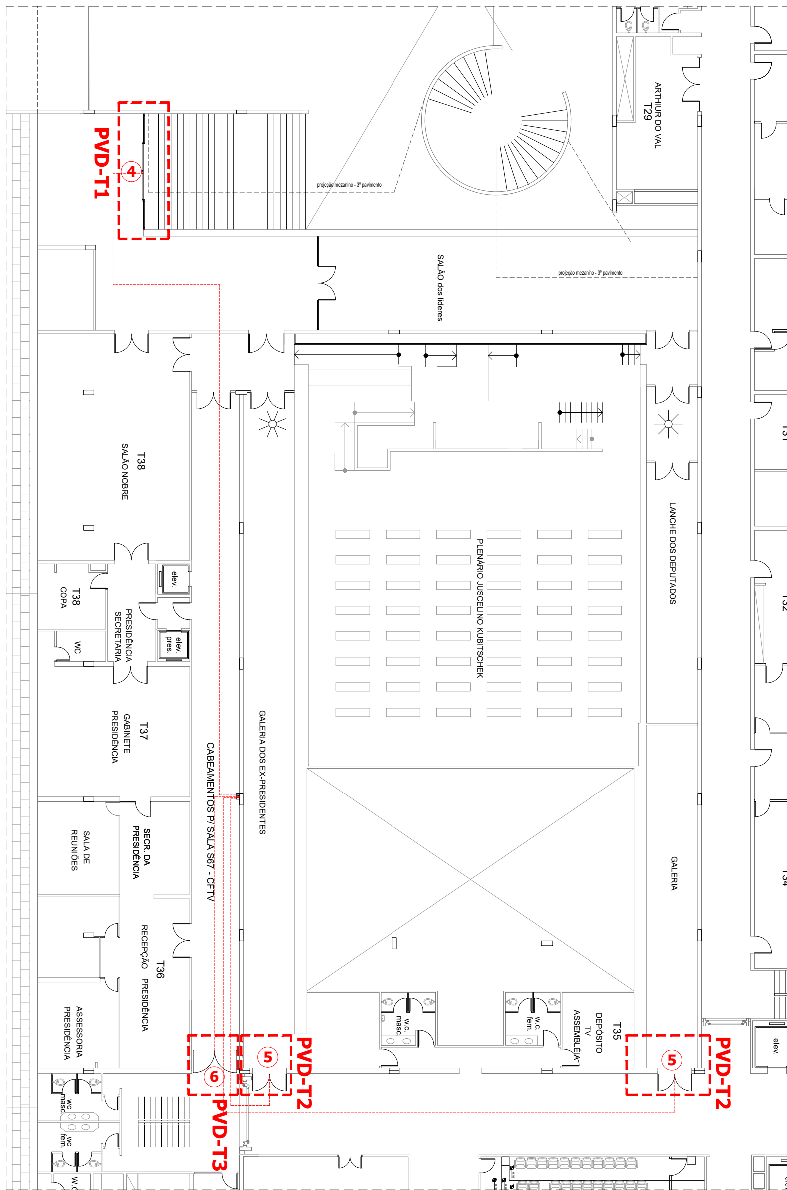
PLANTA ANDAR TERREO
