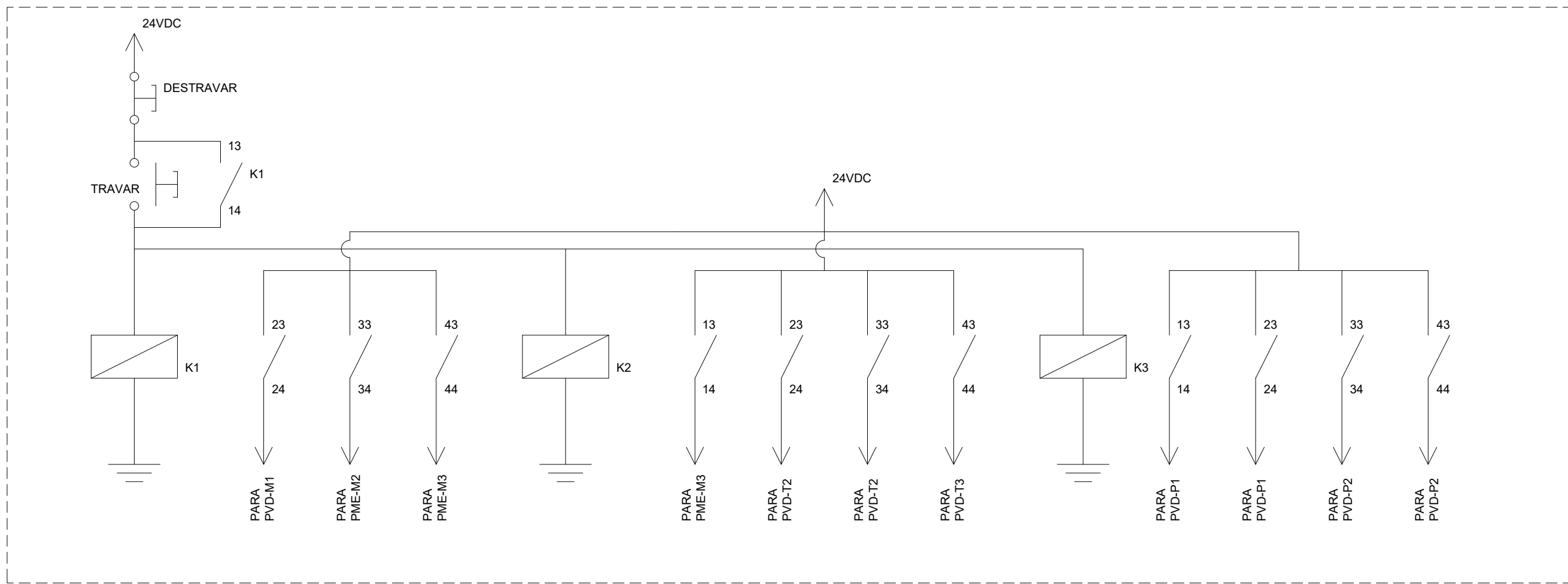
ESQUEMA DE LIGAÇÃO 24V
