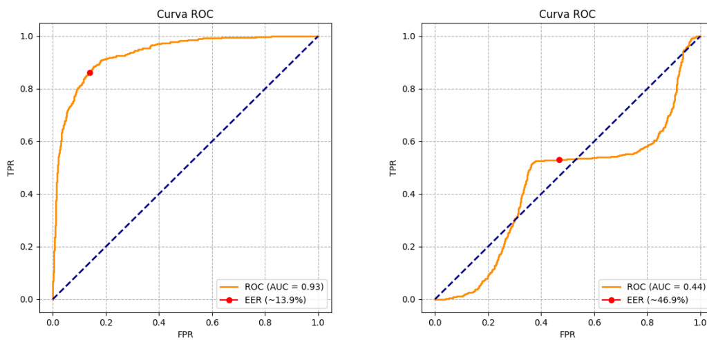
Figura 3 – À esquerda, curva ROC para o CASIA-FASD; à direita, curva ROC do Método 3 treinado no CASIA-FASD e testado no NUAA.
