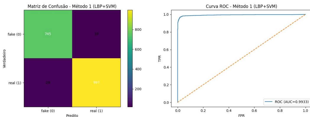
Figura 1 – À esquerda, matriz de confusão; à direita, curva ROC obtida para o Método 1 (LBP + SVM) no conjunto de teste NUAA. As imagens foram geradas pelos scripts de avaliação.
