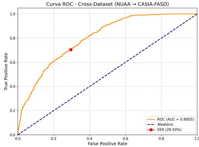
Figura 5 – Curva ROC - CASIA-FASD
