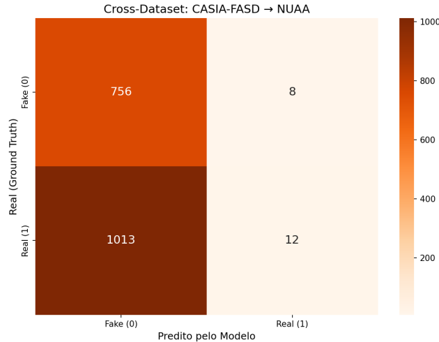
Figura 6 – Matriz de confusão método 2 - CASIA-FASD → NUAA
