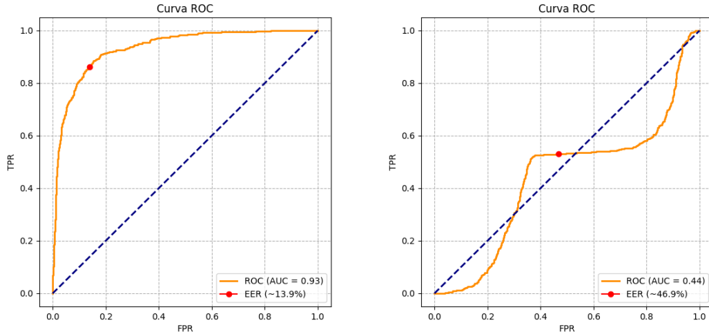
Figura 7 – À esquerda, curva ROC para o CASIA-FASD; à direita, curva ROC do Método 3 treinado no CASIA-FASD e testado no NUAA.
