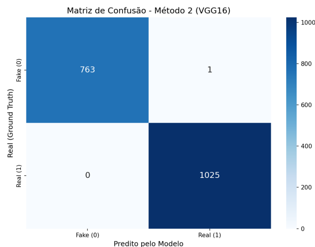
Figura 3 – Matriz de confusão método - NUAA
