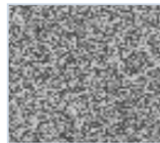
pure noise
