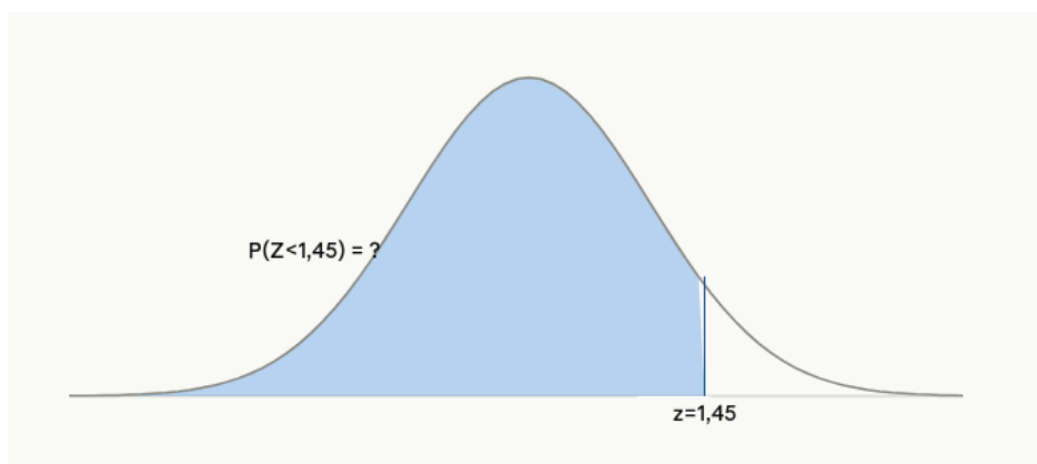
Figura 2.2: Àrea corresponent a P(Z < 1,45) sota la corba normal estàndard.
