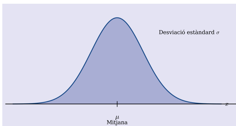
Figura 2.1: Distribució normal amb mitjana \mu i desviació típica \sigma
