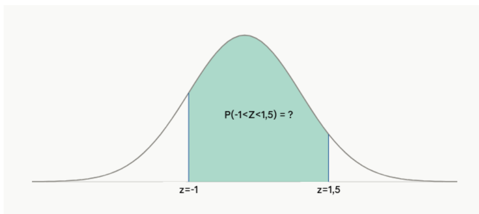
Figura 2.4: Àrea corresponent a P(-1 < Z < 1,5) sota la corba normal estàndard.
