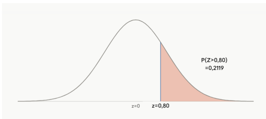
Figura 2.3: Àrea corresponent a P(Z > 0,8) sota la corba normal estàndard.
