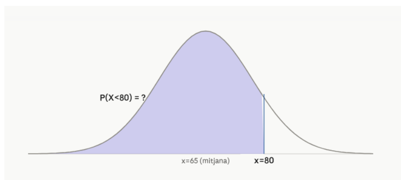
Figura 2.5: Àrea corresponent a X \sim N(65, 12) sota la corba normal estàndard.
