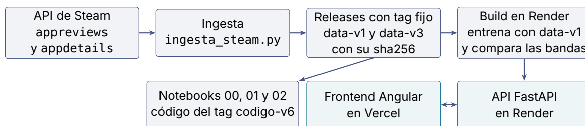
Figura 9: De la API de Steam a la interfaz. Después de la ingestión, ningún paso consulta Steam. Fuente: backend/despliegue/Dockerfile, preparar_entorno.py y frontend/vercel.json.
