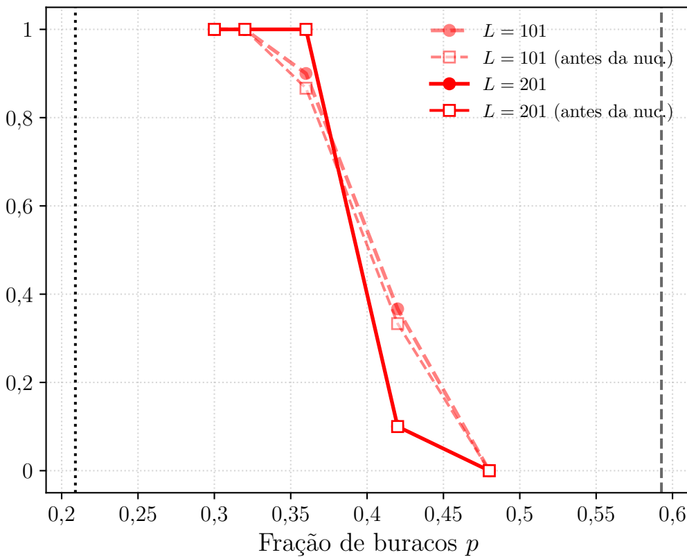
Probabilidade P(\text{escape})
