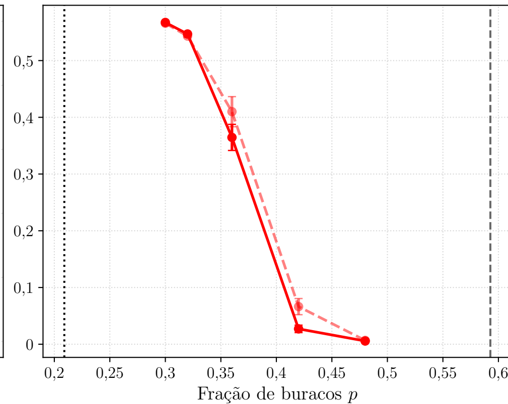
Fração \rho_C estacionária
