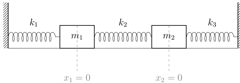
Figura 1: Sistema massa-mola em sua posição de equilíbrio.
