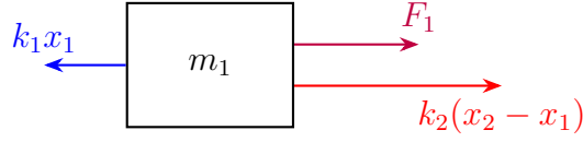
Figura 5: Diagrama de corpo livre para m_1 sujeito a uma força externa F_1 .
