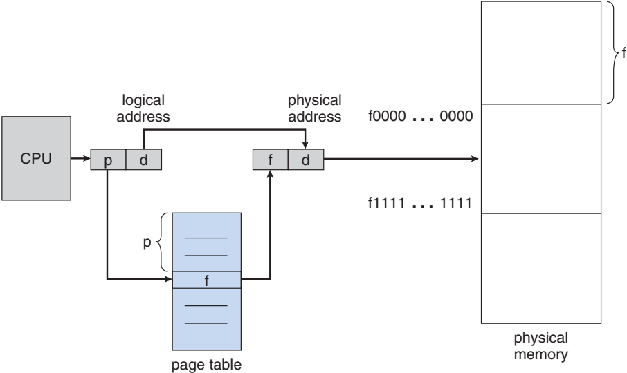
Figure 7.10 Paging hardware.
