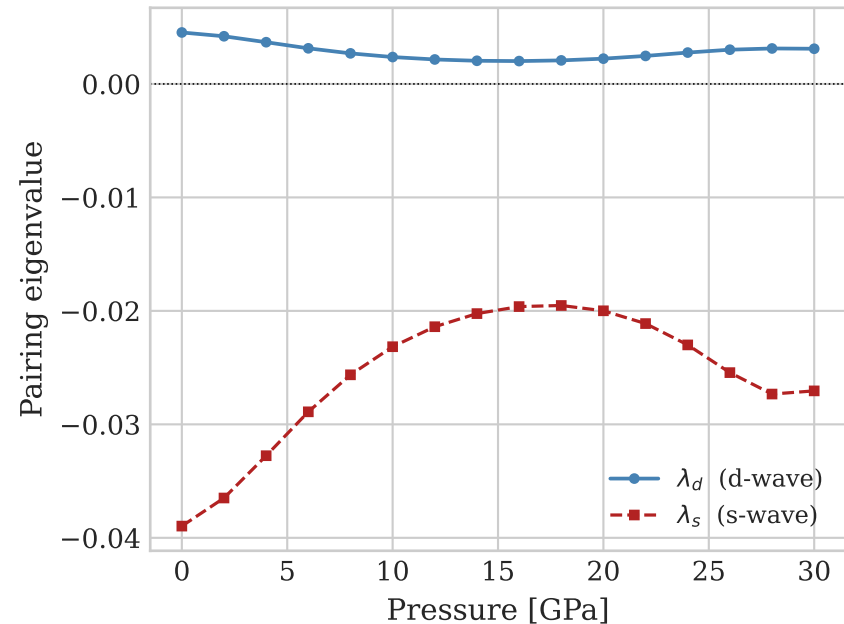
RPA channel eigenvalues
