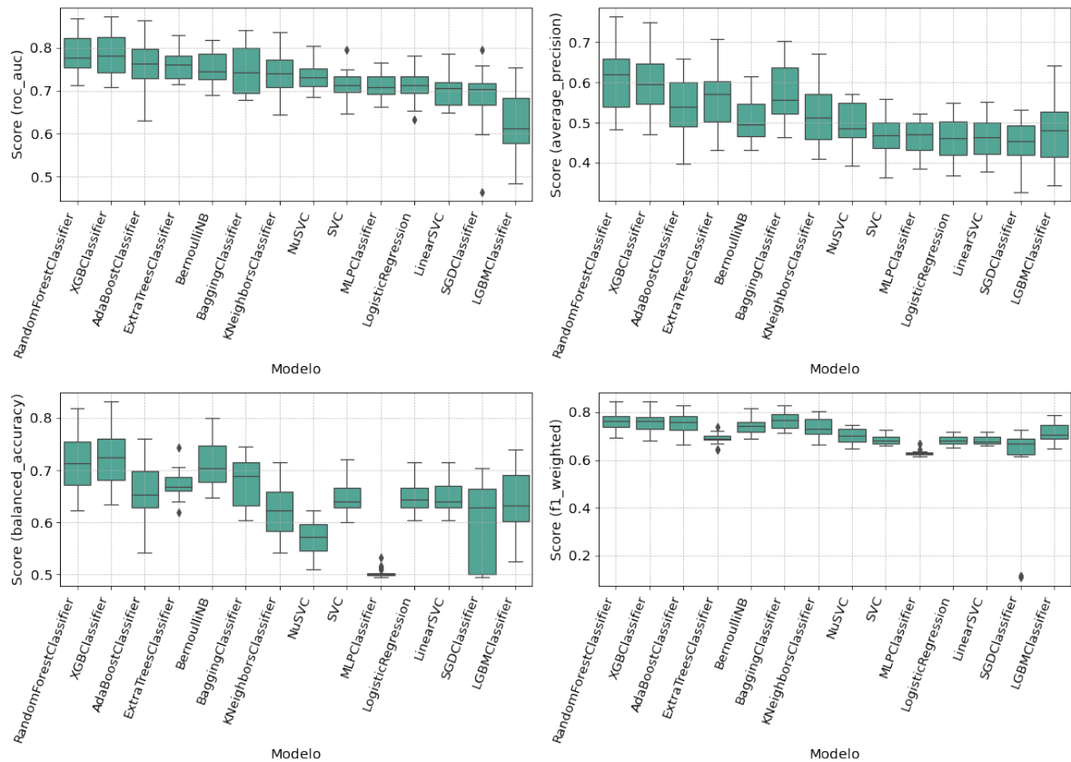
Figura 6 – Distribuição dos scores por métrica e modelo
