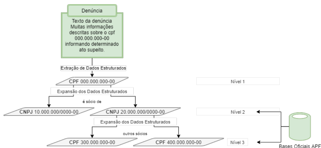
Figura 3 – Exemplo de extração e expansão de dados estruturados
