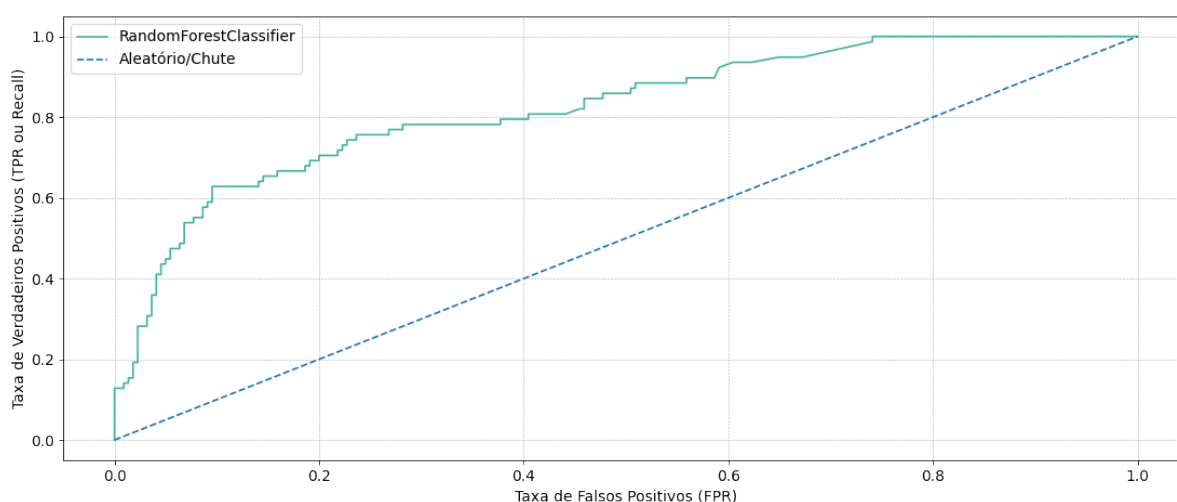
Figura 7 – Curva Característica de Operação do Receptor (ROC)
