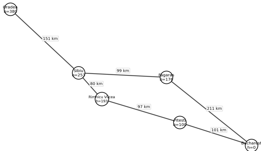
Subgrafo relevante: Oradea → Bucharest
