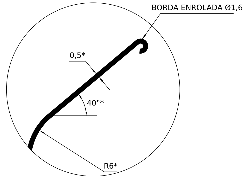
DETALHE A ESCALA 5:1
