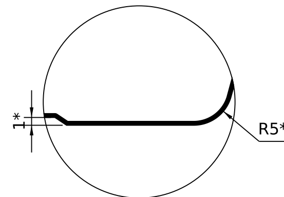
DETALHE B ESCALA 2:1
