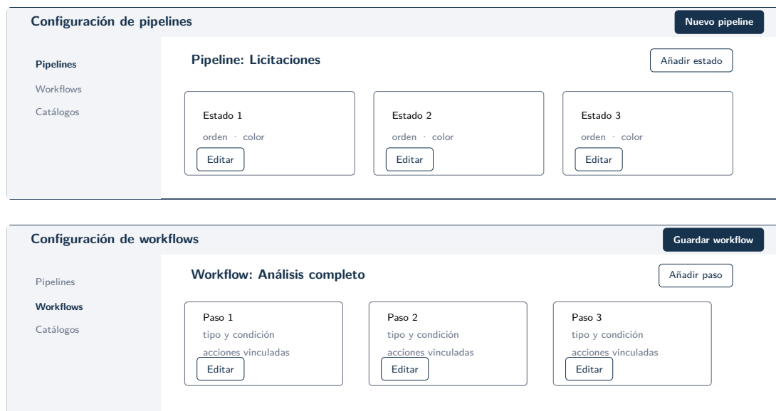
Figura 4.18: Wireframes de configuración de pipelines y workflows.
