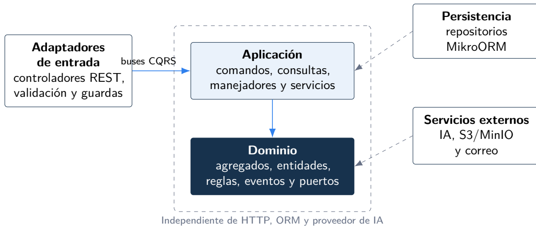
Figura 5.2: Capas, puertos y adaptadores del backend.
