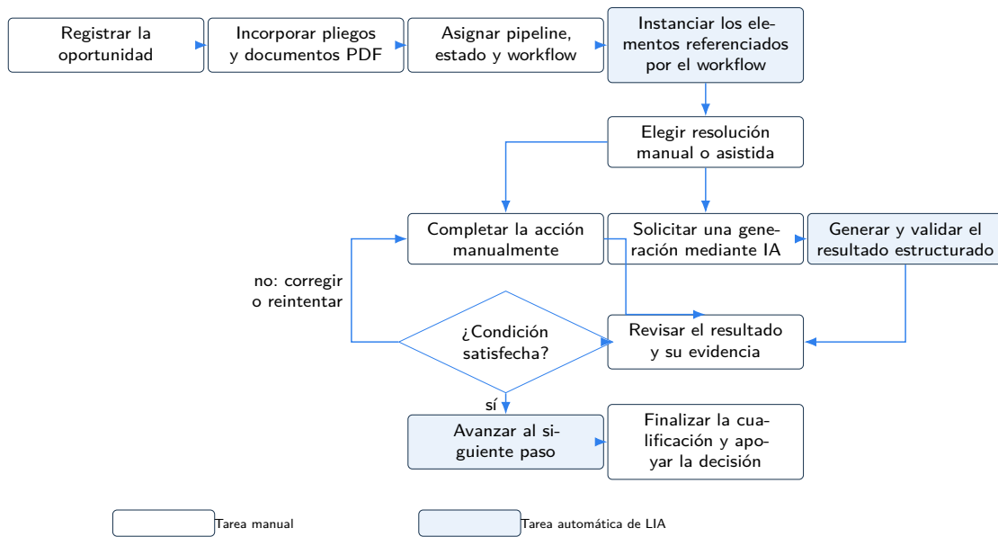
Figura 4.3: Proceso de cualificación con tareas manuales y automáticas.
