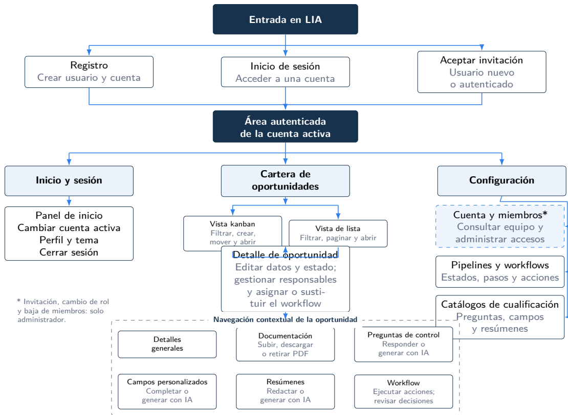
Figura 4.8: Diagrama de navegabilidad propuesto para LIA.
