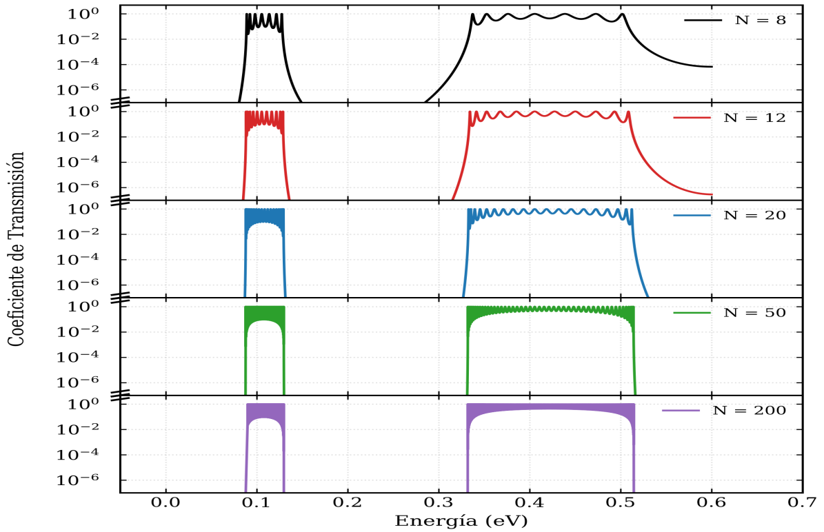
Figura 4: Formación e individualización de la minibanda de conducción en ejes apilados.
