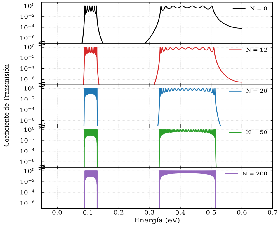
Figura 4: Formación e individualización de la minibanda de conducción en ejes apilados.
