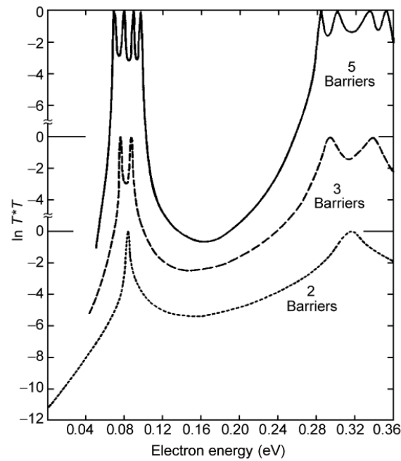
Figura 4: Resultados de Tsu y Esaki ([8]) para una red de 5 barreras con parámetros similares a los nuestros.
