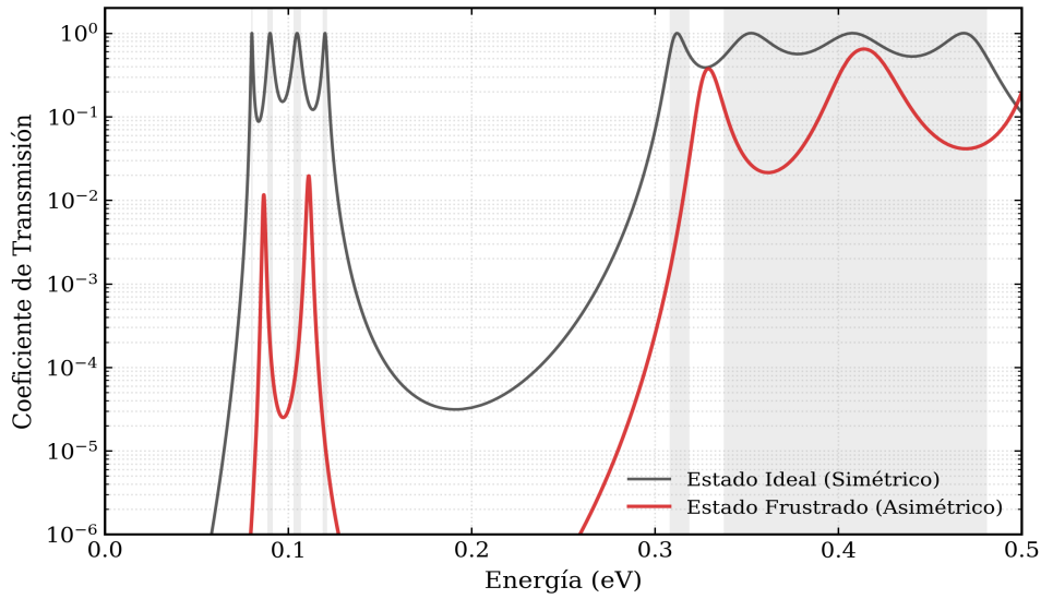
Figura 5: Efecto de la frustración por desalineación energética (célula mutada de 10 nm).
