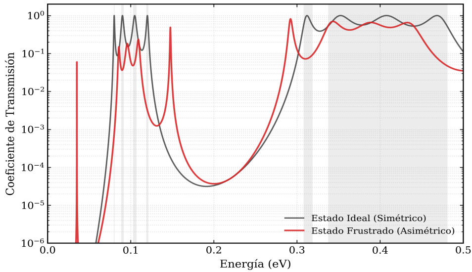
Figura 6: Efecto de la frustración por bloqueo de interfase (septo calcificado de 8 nm).
