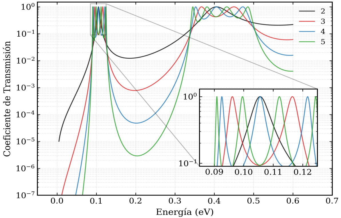
Figura 1: Coeficientes de transmisión solapados con recuadro de zoom ( N = 2 a 5 ).
