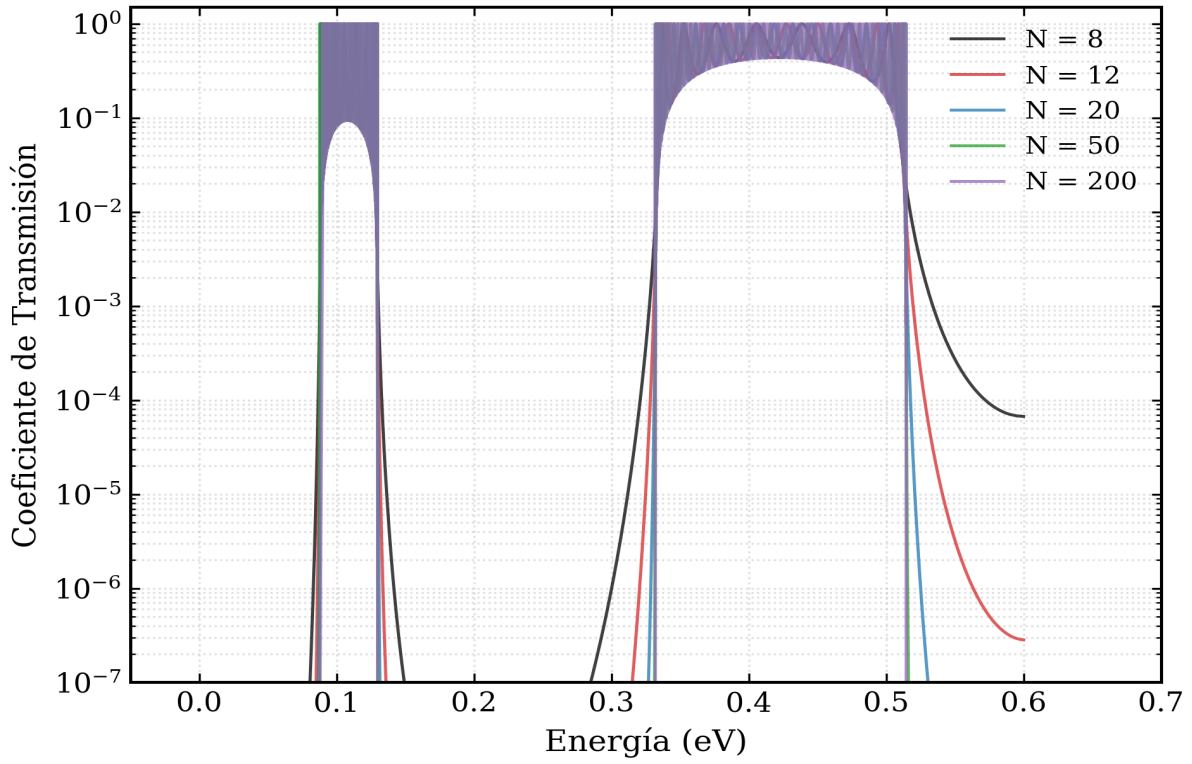
Figura 3: Evolución macroscópica hacia el continuo sólido de bandas ( N = 8 a 200).
