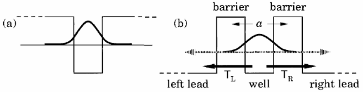
Figura 1: Comparación entre barreras infinitas y barreras finitas [3].
