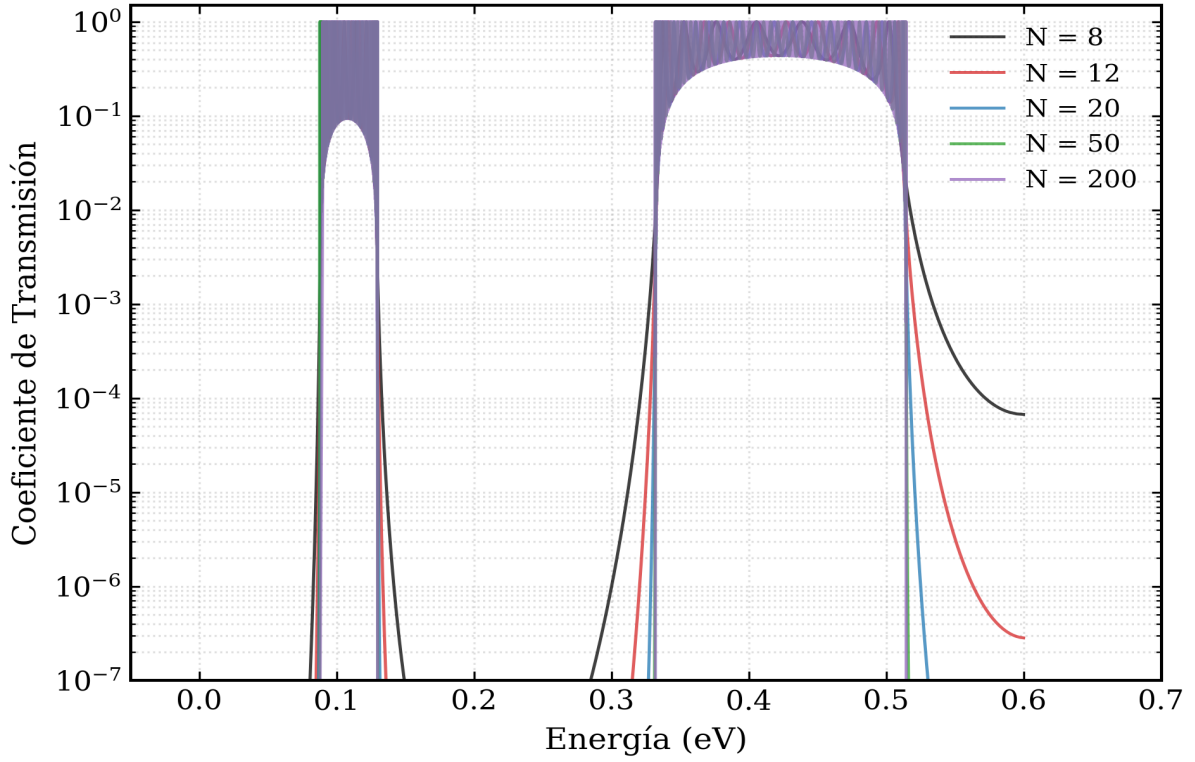
Figura 4: Evolución macroscópica hacia el continuo sólido de bandas ( N = 8 a 200).
