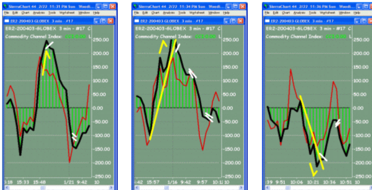
Три графика выше - Паттерн "Экстремальный Крюк (HFE)".
