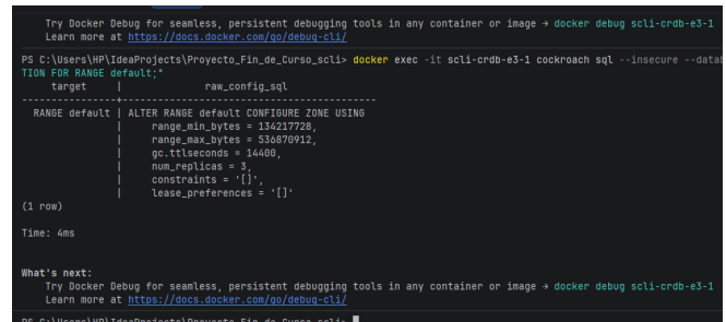
Figura 8: Configuración de zona del rango default, con num_replicas = 3 aplicado.
