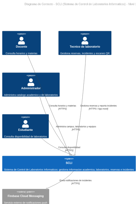
Figura 2: C4 Nivel 1 – Contexto del sistema SCLI
