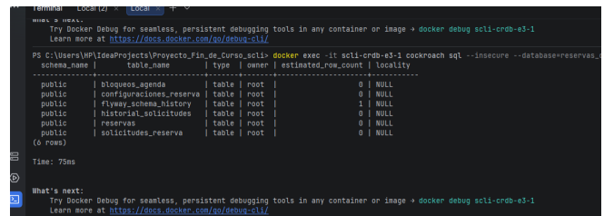
Figura 7: Tablas del esquema reservas_db aplicado en el clúster E3.
