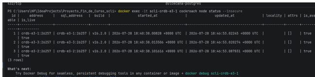
Figura 6: Estado de los tres nodos del clúster E3 ( cockroach node status ): los tres reportan is_live=true .
