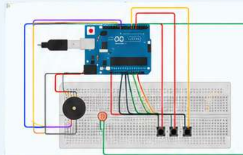
Prototipo funcional de IRTRA StormSafe en Tinkercad.
