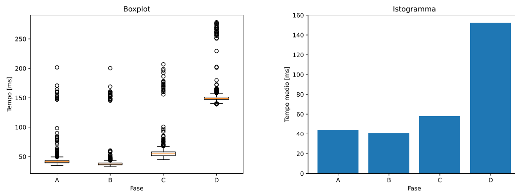
Figura 5.2: Boxplot e istogramma relativi ai tempi di esecuzione dell'applicazione a microservizi
