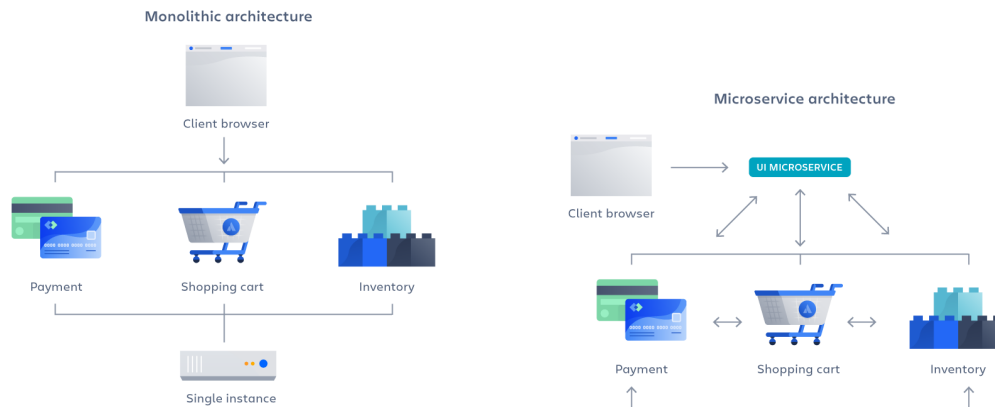
Figura 2.1: Principio di funzionamento di un'applicazione monolitica e una a microservizi[10]
