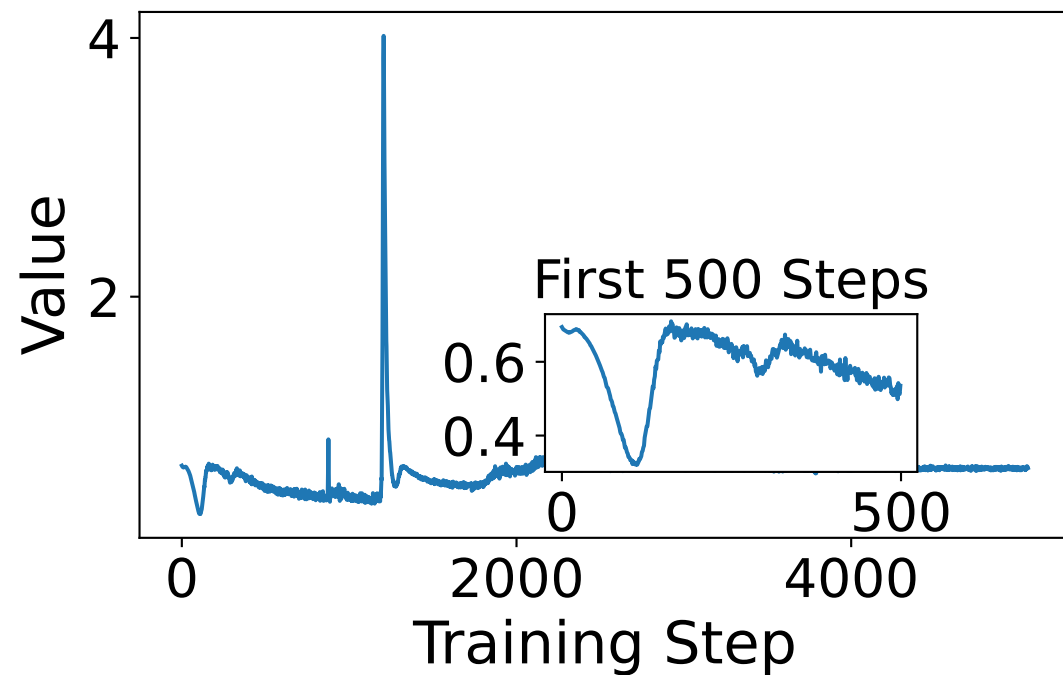
Generator MSE
