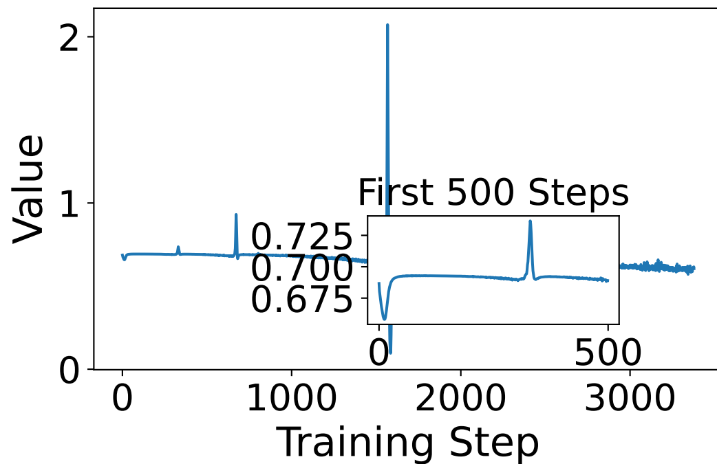
Generator MSE
