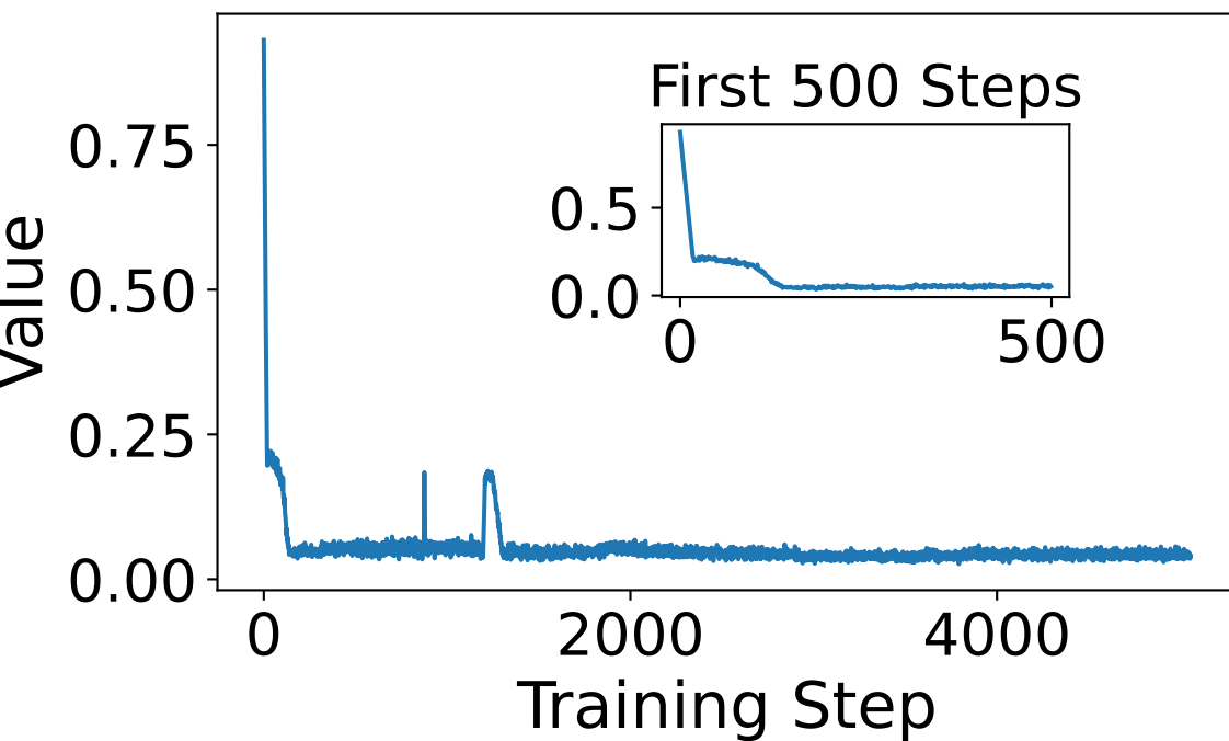
Generator MSE
