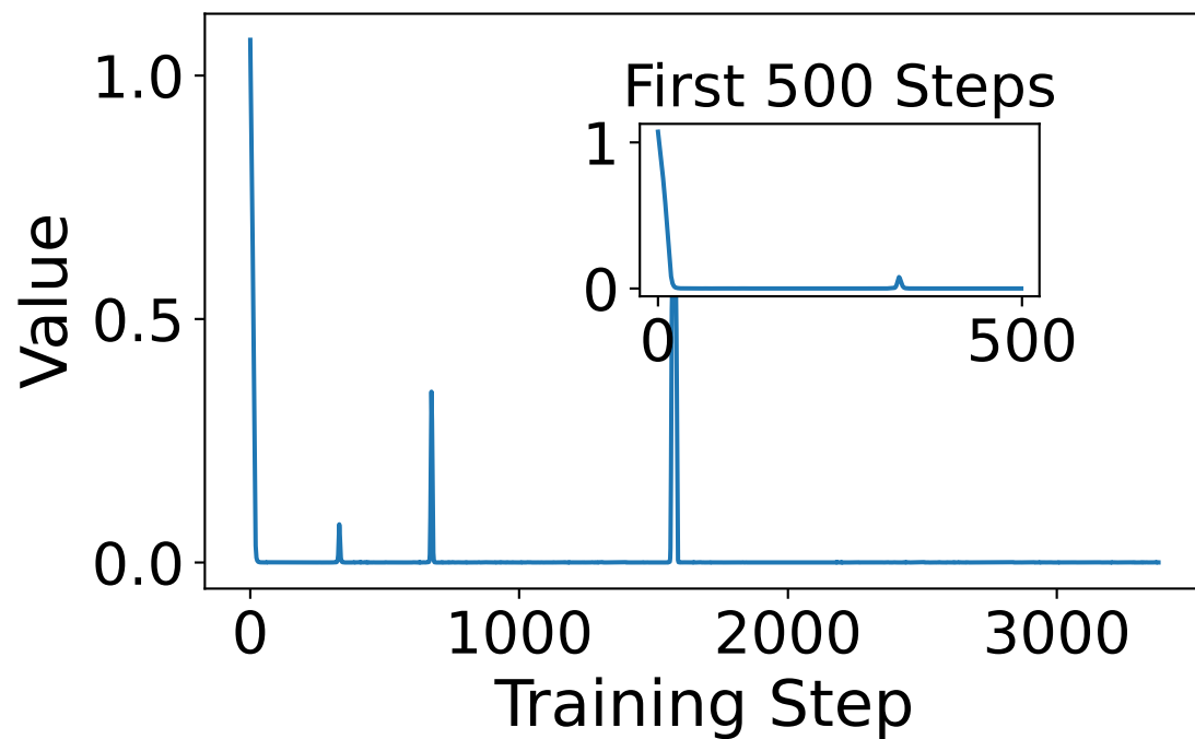
Generator MSE
