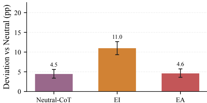
GPT-5
