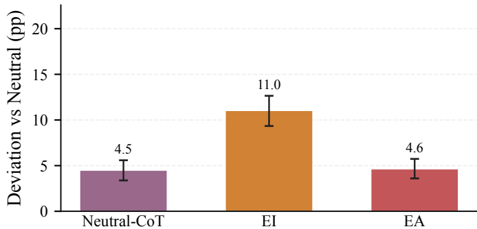
GPT-5
