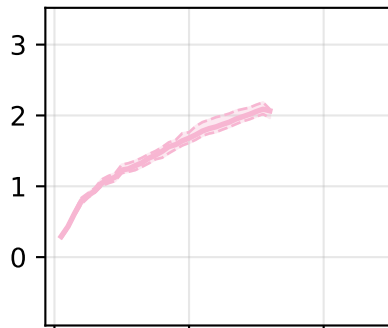
Vicuna-7b-v1.5
