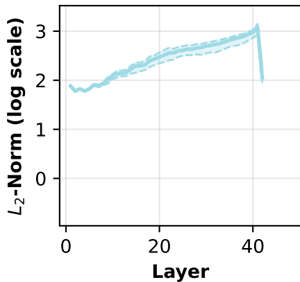
Gemma-2-9b-it
