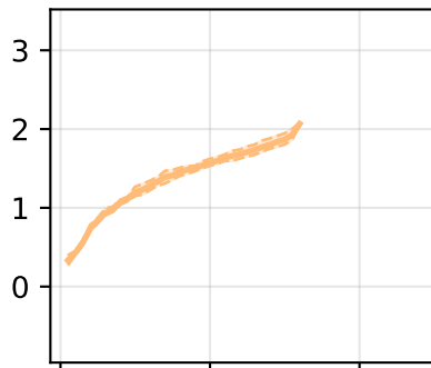
Vicuna-7b-v1.5
