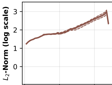
Gemma-2-9b-it
