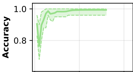
Mistral-SU
