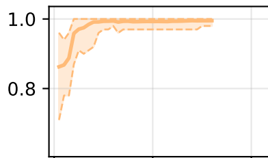
Llama3-LAT
