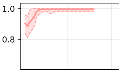
Llama3-TAR
