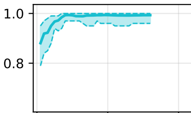
Llama3-RB
