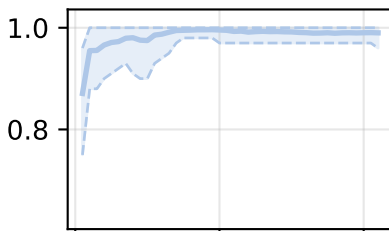
Gemma-DA
